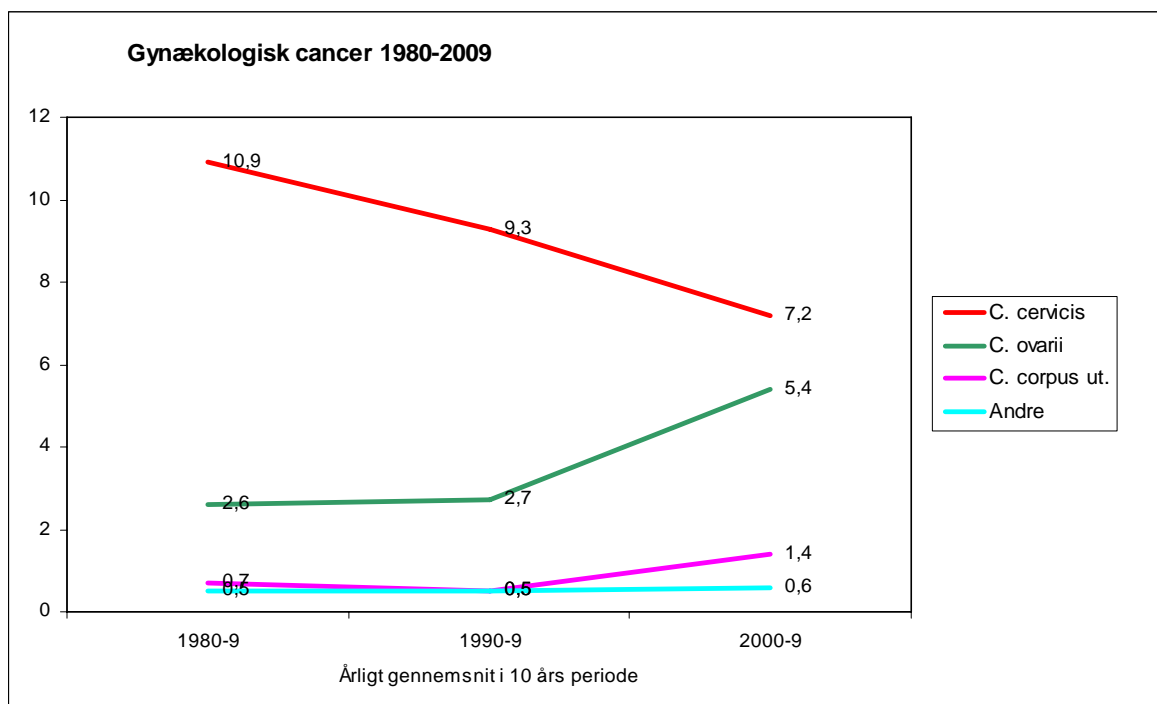
Titartagaq 6.7: 1980-imiit 2009-p tungaanut illissap paavatigut kræfteqartut (livmoderhalskræft (c. cervicis), mannessaqarfikkut kræfteqartut (c. ovarii) aammalu illissakkut kræfteqartut (c.corpus uteri) 1980-2009. Ukiut qulit ingerlaneranni ukiumoortumik agguaqatigiissitsineq
