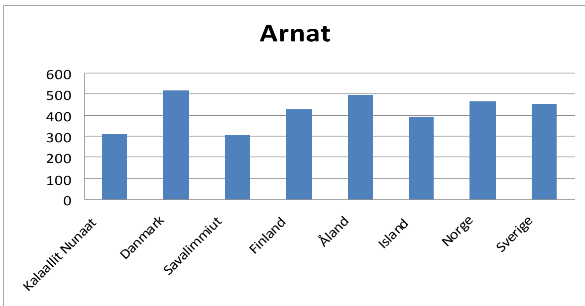
Titartagaq 2.6 2000-mit 2004-mut nunani avannarlerni arnat akornanni kræftimik nappaateqaleqqartutut paasisaqarfioqqaartut, angutinu 100.000-ikkaanut "nordisk standardpopulation"-imilu aallaavigalugu naatsorsukkat (NOMESCO-mit paasisutissiissutit)
